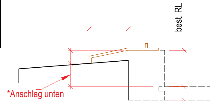
Seitenriss unten
